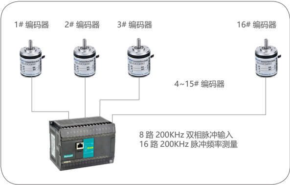
Haiwell PLC 带 16 个编码器
